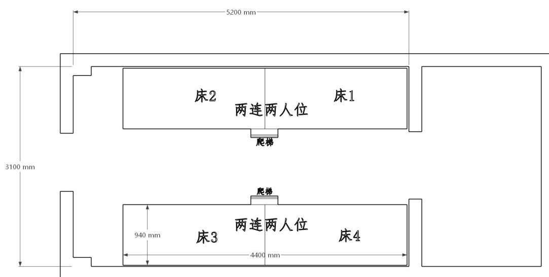
平面布置图（四人间加长床）
