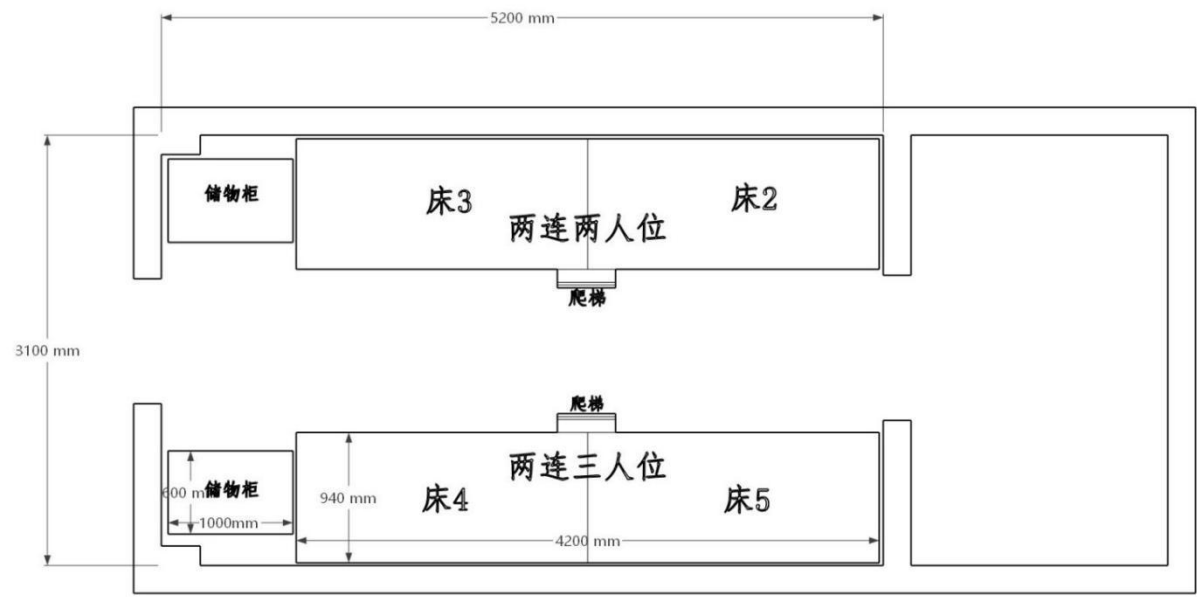
平面布置图（五人间）
